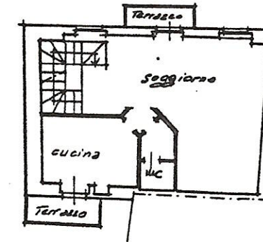
Piano Secondo H=2.43
